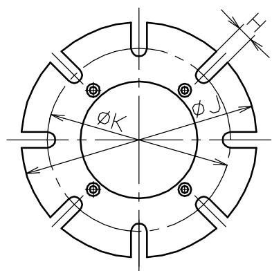
MGF-202 フランジ
