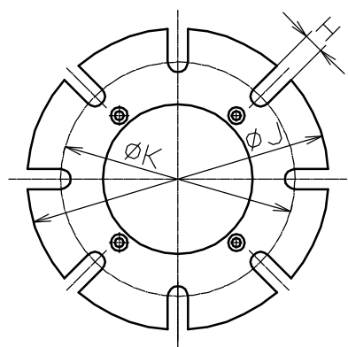
MGK-82,152 フランジ
