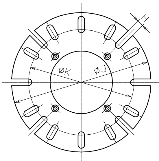
MGK-192 フランジ
